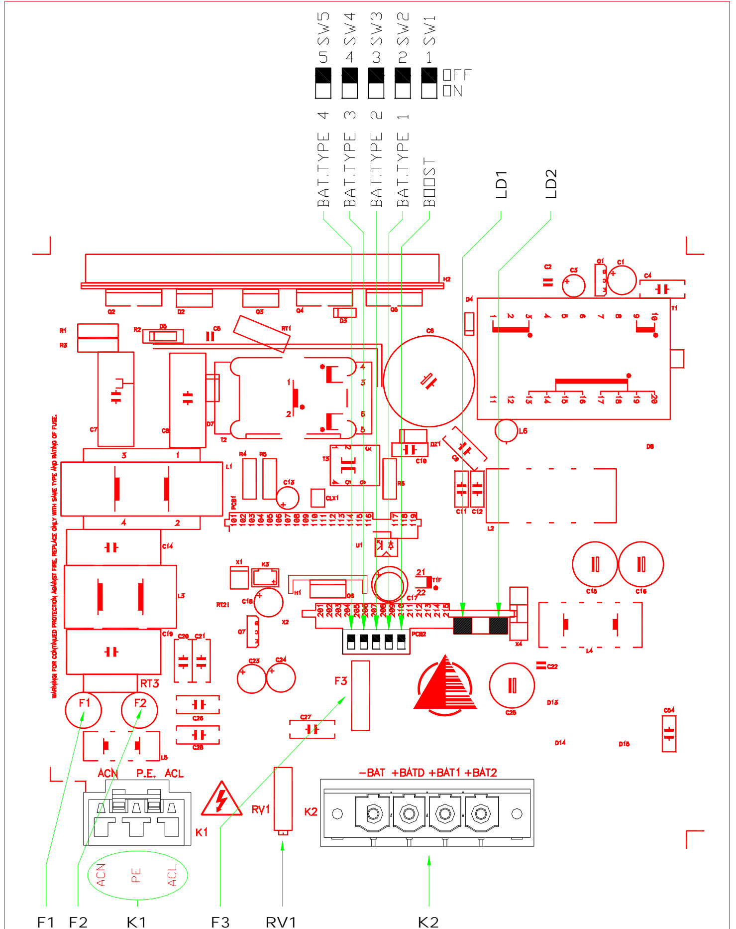
Carte chargeur / Charger board / Ladegerätkarte / Tarjeta cargador / Scheda caricatore / 12V/25A 13-03-2006 N°09042 10A
