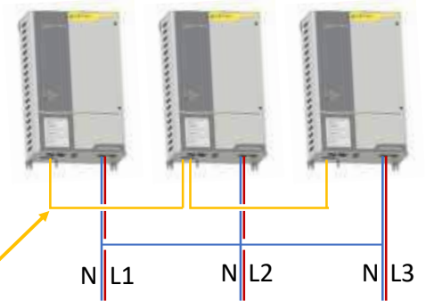
Montage triphasé
